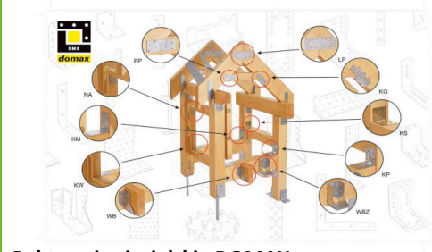
Połączenia ciesielskie DOMAX
