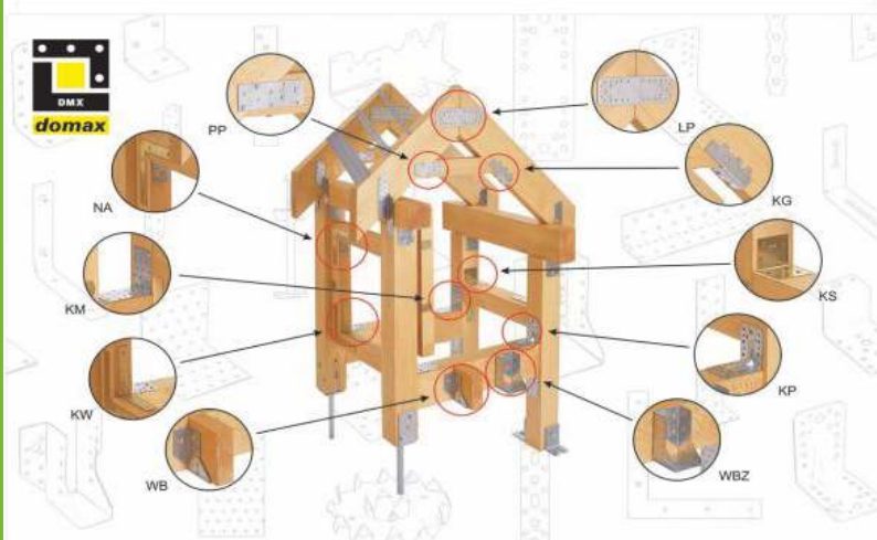
Okucia ciesielskie DOMAX
