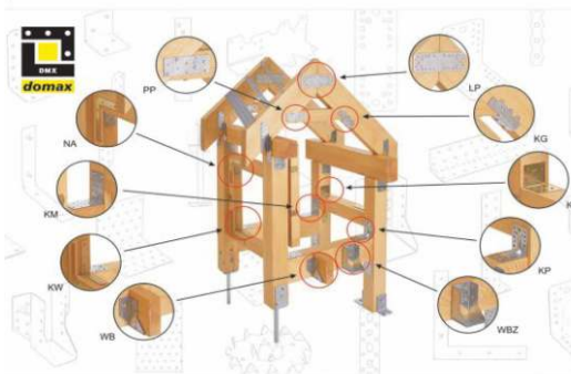
Okucia ciesielskie DOMAX
